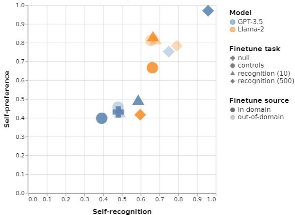
CNN/Dailymail
